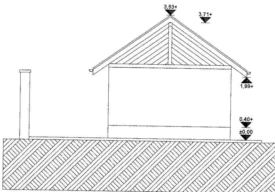
H11-H11 HOMLOKZAT
