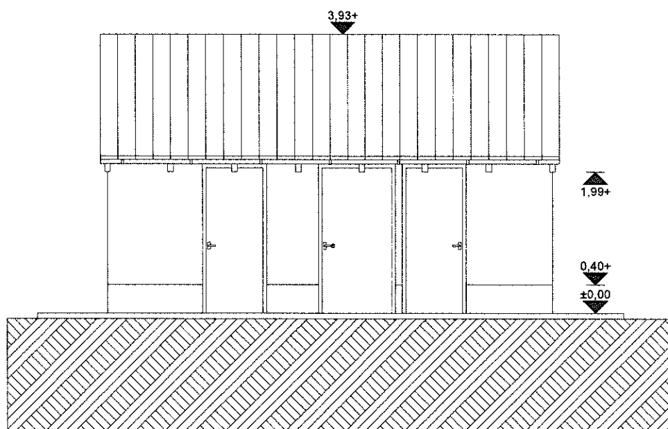
H12-H12 HOMLOKZAT
