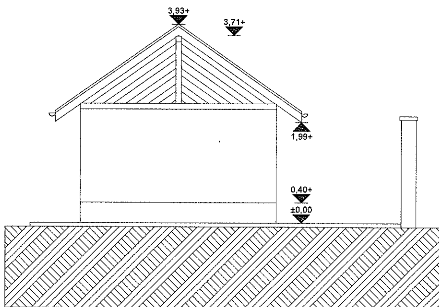
H13-H13 HOMLOKZAT
