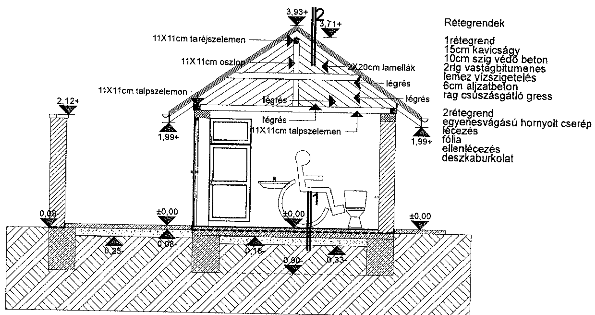
A1-A1 METSZET
